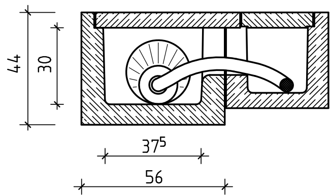
Systemschnitt
