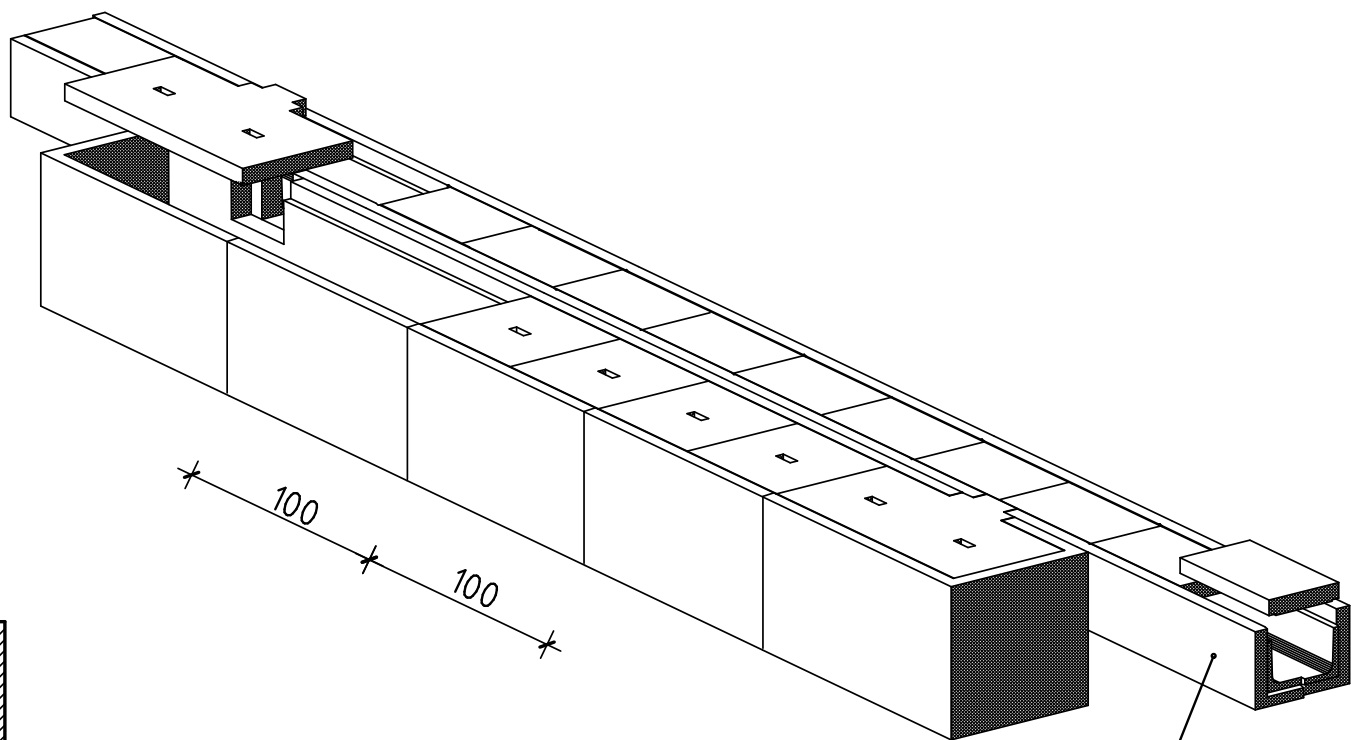
Ausführung IIIa
