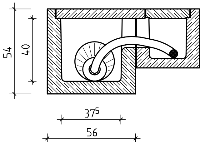
Systemschnitt
